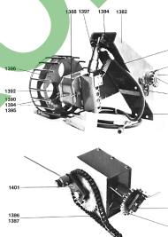
ETB-011541, Akcesoria specjalne: napęd od koła jezdnego
