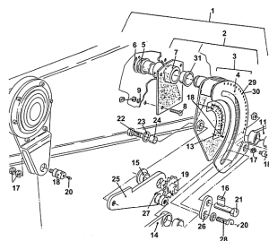
ETB-011543, Bezstopniowa regulacja dawki
