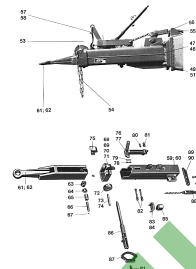
ETB-011505, Rama: dyszle
