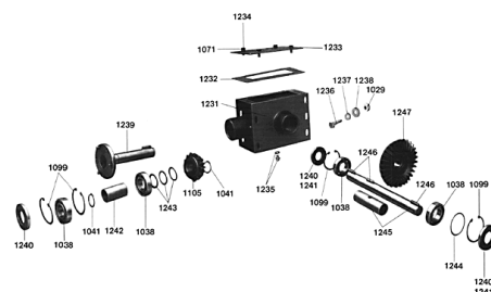
ETB-011536, Akcesoria specjalne: ślimak rozsiewający (przekładnia)
