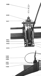
ETB-011542, Podwozie: hamulec hydrauliczny
