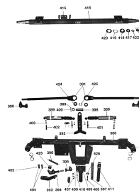
ETB-011513, Podwozie: oś tandemowa (tylna i przednia oś
