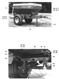
ETB-011504, Rama: rama, płyta denna, szybkozłącze mechanizmu rozsiewającego
