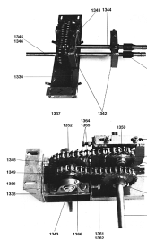
ETB-011540, Akcesoria specjalne: napęd 540 / 100 obr./min
