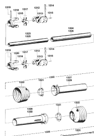
ETB-011539, Napęd: wałki przekładnikowe (WI-UC 12)
