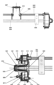
ETB-011511, Podwozie: oś (oś hamowana StA 8X, rozstaw kół
