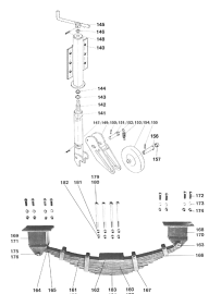
ETB-011507, Podwozie: koło podporowe, zawieszenie
