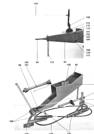
ETB-011506, Rama: dyszle (wałek przekątnikowy, dźwignia hamulca)
