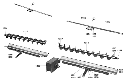
ETB-011535, Akcesoria specjalne: ślimak rozsiewający (korytko rozsiewające)
