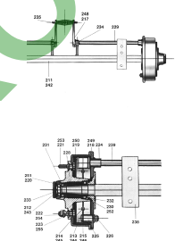
ETB-011509, Podwozie: oś (oś hamowana StA 8, rozstaw kół 1700 mm; 5,7 t i 1740 mm; 4,2 t)
