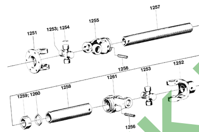
ETB-011537, Akcesoria specjalne / napęd: ślimak rozsiewający (wałek przekładnikowy)
