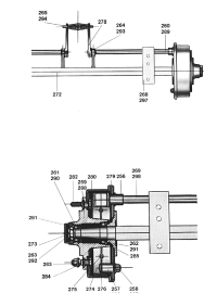
ETB-011510, Podwozie: oś (oś hamowana StA 10, rozstaw kół 1850 mm; 7,5 t)
