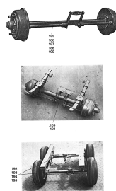
ETB-011508, Podwozie: oś hamowana, oś tandemowa hamowana)
